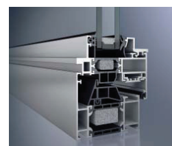
Schüco Ventana AWS 70 ST.HI sistema con contorno estrecho de acero Schüco Window AWS 70 ST.HI system with narrow steel contour
